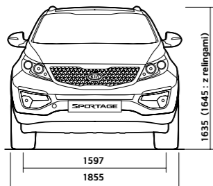
Wymiary zewnętrzne (mm)
